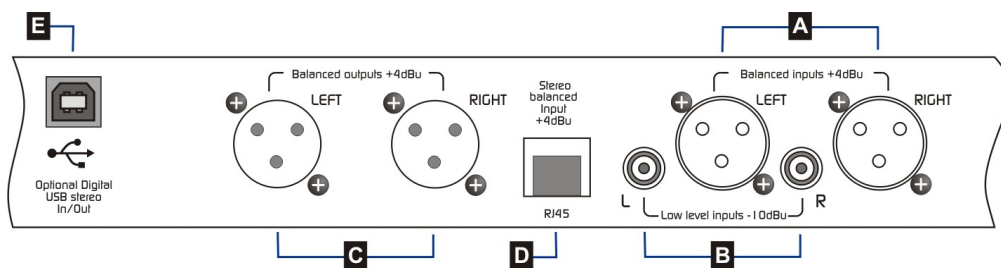
entradas y salidas analógicas en el panel trasero
